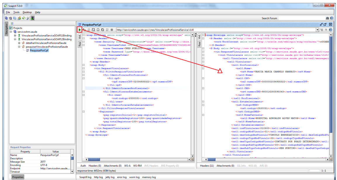
Figura 12: XML padrão da resposta (response).
